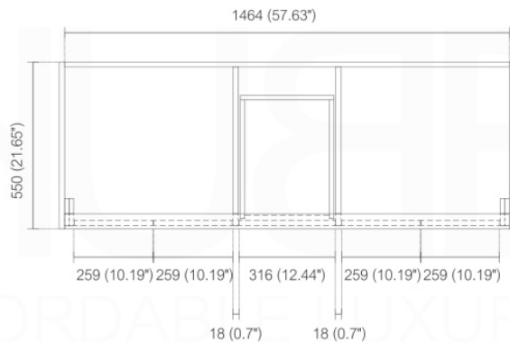
. TOP ELEVATION
