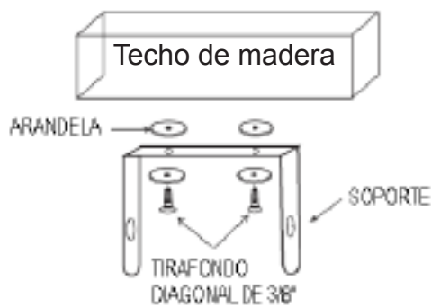
Figura 4b. Montaje de dos tornillos
