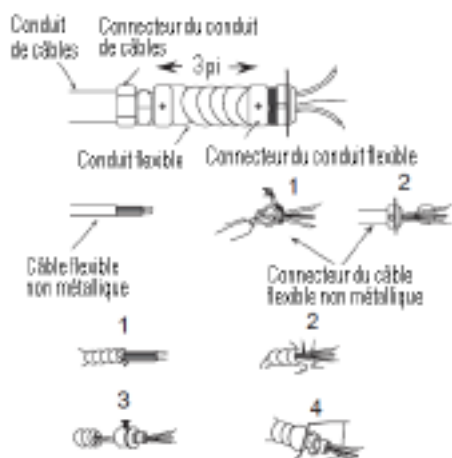
Figure 6 – Connecteurs, câbles et quincaillerie utilisés pour brancher le radiateur
