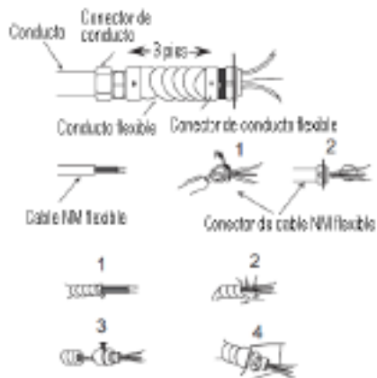
Figura 6. Conectores, cable y demás elementos utilizados para el cableado del calefactor
