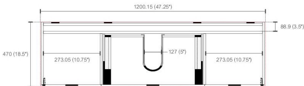
. TOP ELEVATION
