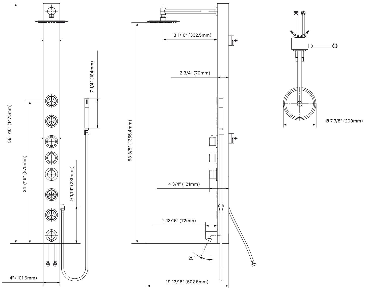
Top View / Vista Superior / Vue de Dessus
