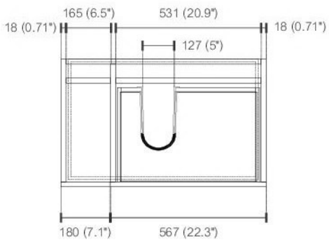
TOP ELEVATION
