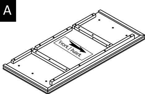
TOP QTY 1
