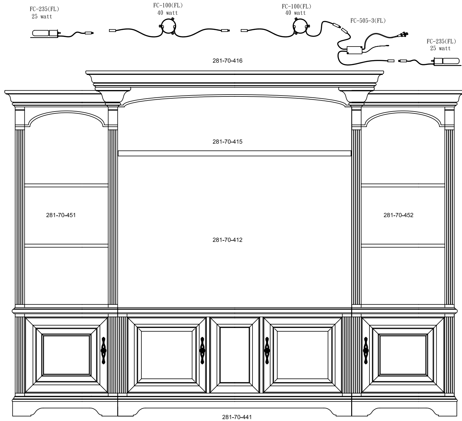
281-70-燈連接示意圖
