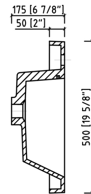
SECTION A-A
