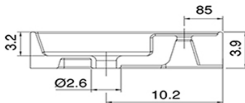
SEZIONE A-A
