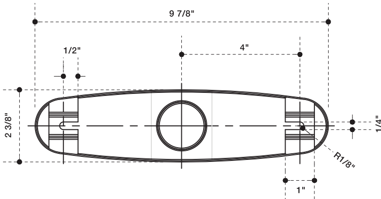
BOTTOM VIEW VISTA DE FONDO VUE DE DESSOUS
