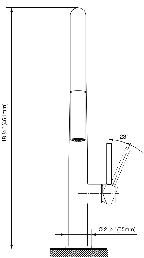
SIDE VIEW / VUE DE CÔTÉ / VISTA LATERAL
