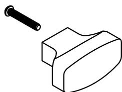
HANDLE a. M4 X 25 mm - QTY2 b. M4 X 35 mm - QTY1 QTY 3 SETS
