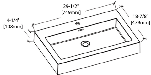
TOPMOUNT (A10 3019 04)
