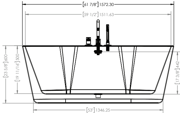
FRONT VIEW VUE DE FACE
