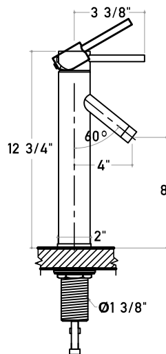
SIDE VIEW VUE DE CÔTÉ VISTA LATERAL
