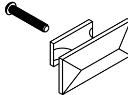
HANDLE M4 X 30 mm QTY 6 SET
