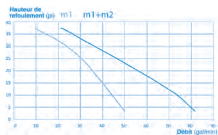
Courbe de débit SANICUBIC® 2
