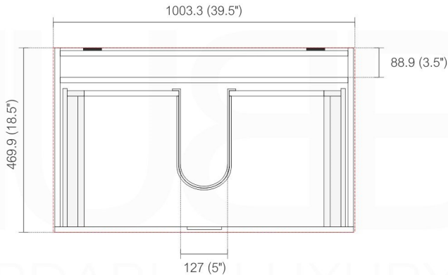
. TOP ELEVATION
