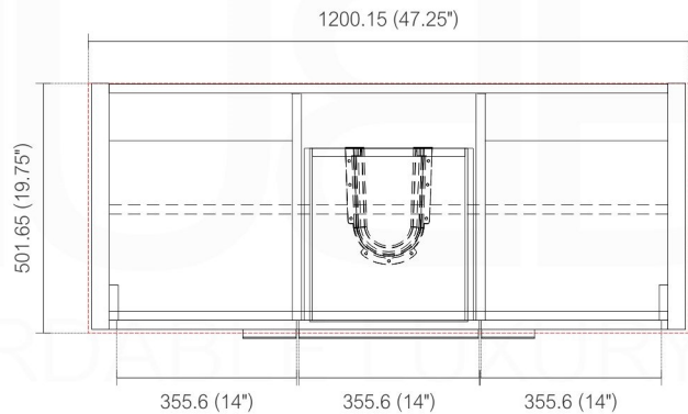
. TOP ELEVATION
