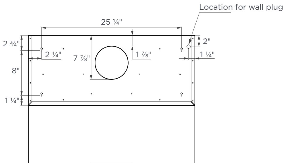
TOP
