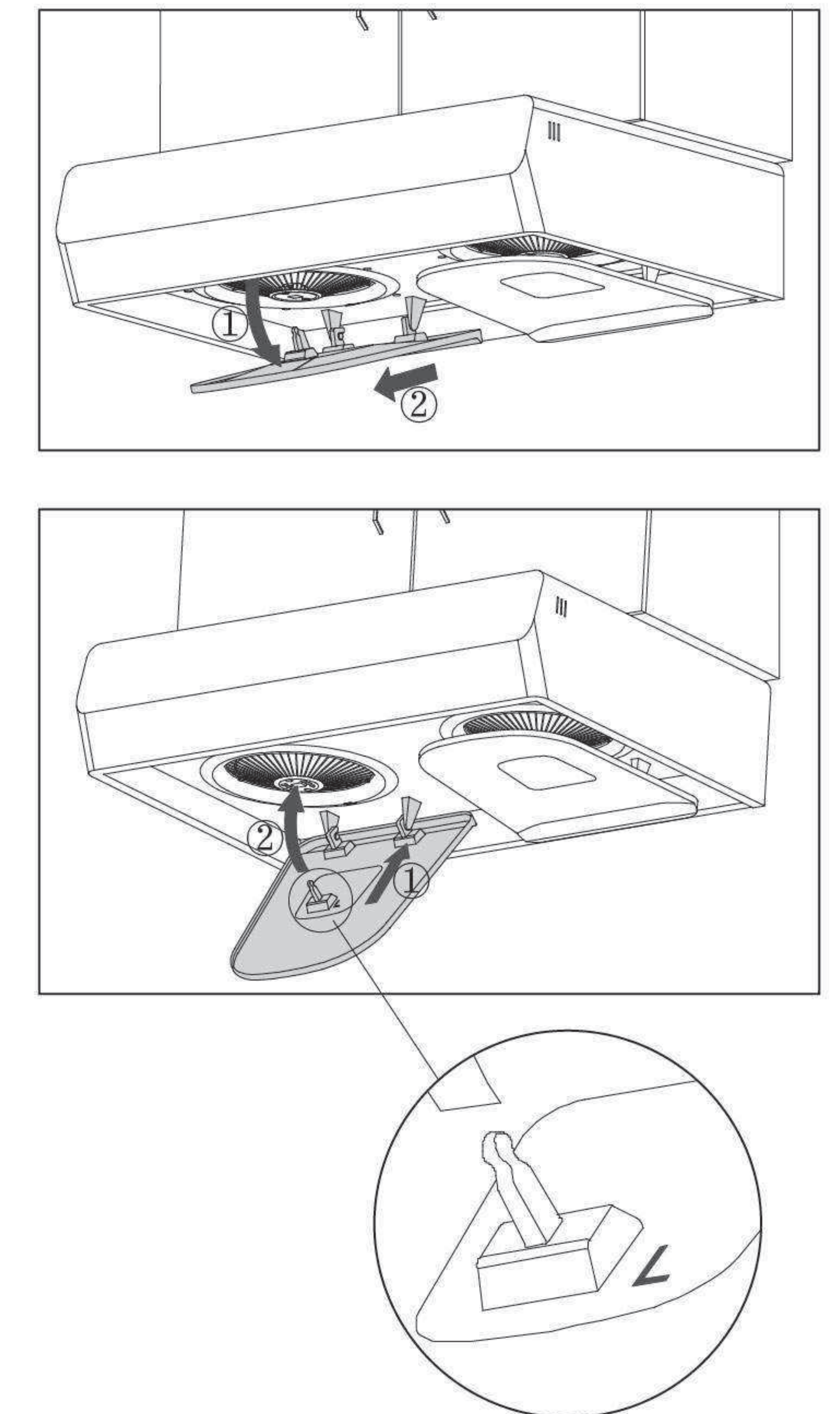
Diagrama esquemático de desmontaje y montaje del panel de ala de mariposa (aceitera integrada)
