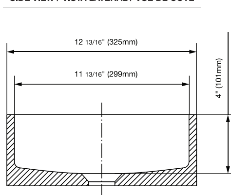
SIDE VIEW / VISTA LATERAL / VUE DE CÔTÉ
