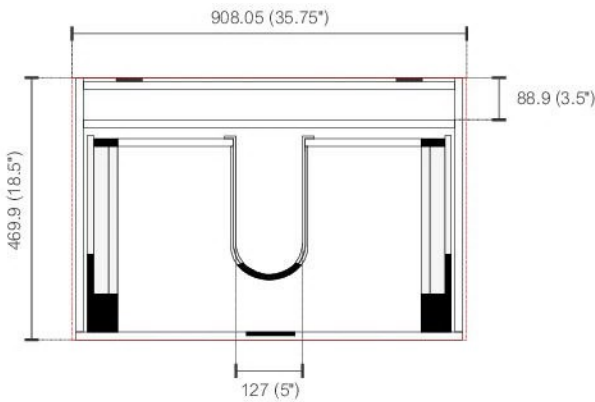
. TOP ELEVATION
