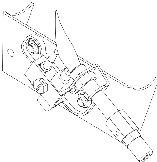
Fig. 21 - Patrón incorrecto de llama piloto
