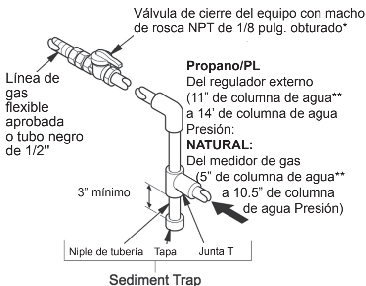
Fig. 10 - Conexión del gas
