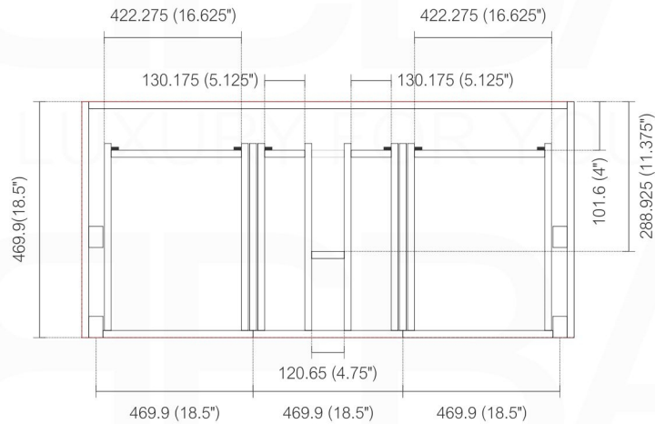
TOP ELEVATION
