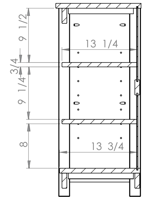
SEÇÃO A-A
