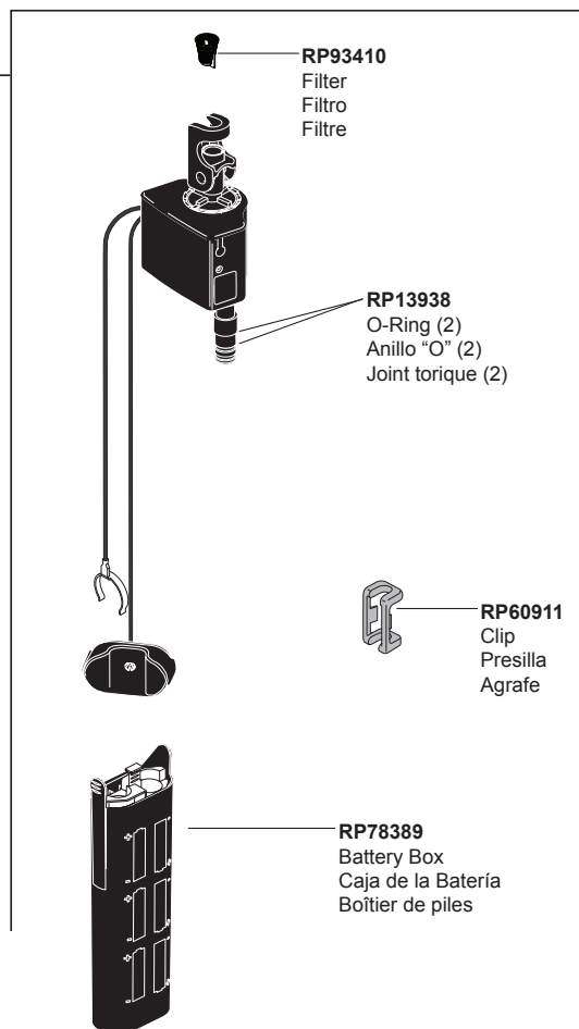
EP74855 Solenoid Assembly Ensemble de Solenoïde Électrovanne For PC & SS finishes, order EP74855 For SP finishes, order EP74855XX Para acabados PC y SS, ordene EP74855 Para acabados SP, ordene EP74855XX Pour les finis PC et SS, commandez EP74855 Pour les finis SP, commandez EP74855XX
