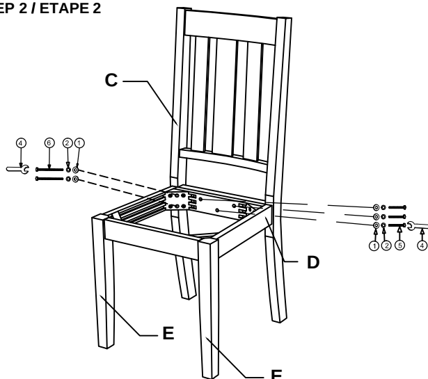
STEP 2 / ETAPE 2
