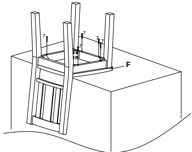
STEP 4 / ETAPE 4
