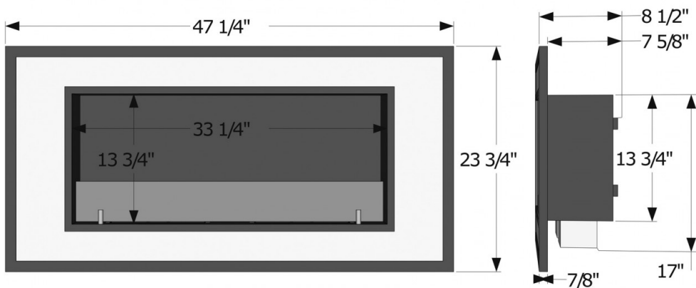
Bellezza Fireplace Dimensions
