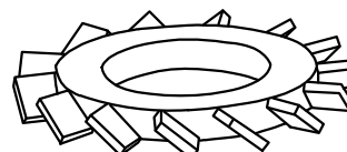
LOCK WASHER Ø15 / Ø8 X 2 mm QTY 8
