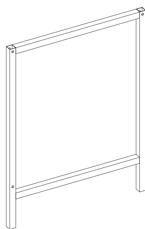
A:Desk Leg Frame, Left 1PC
