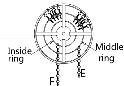
Fig 1.1 Round frame(D)
