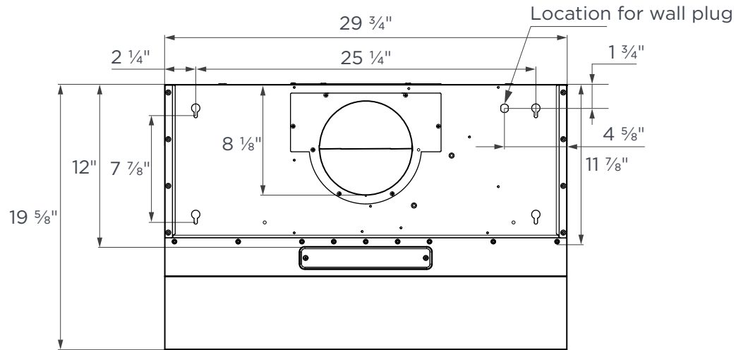
TOP
