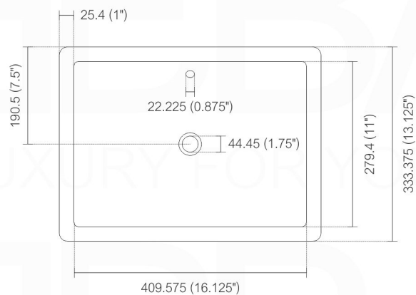
TOP ELEVATION
