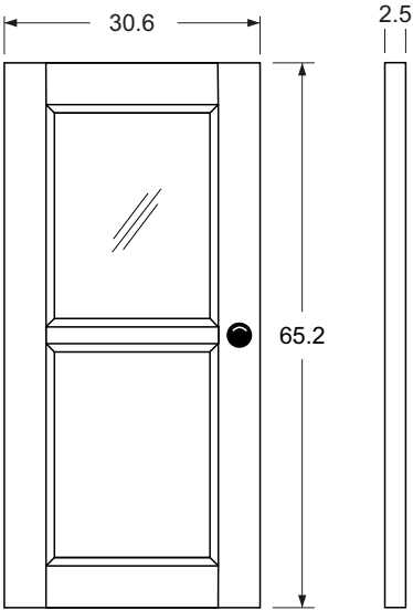
DOOR DETAIL
