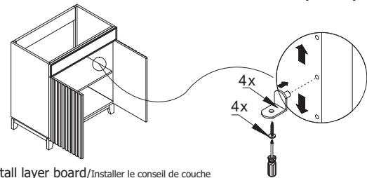
1. Install layer board/Installer le conseil de couche
