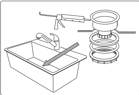
Install Drain with Silicone Sealant Instalar el drenaje con sellador de silicona
