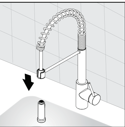
Remove Sprayer Quitar pulverizador
