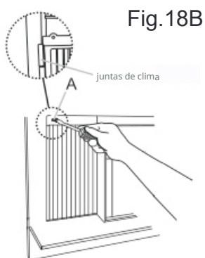
A. Tornillo hexagonal largo de 3/4 (o 1/2) pulgada
