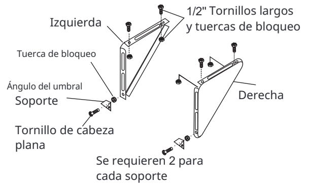
Fig. 15B
